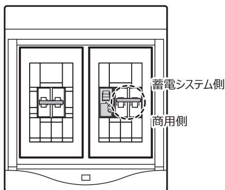
蓄電出力切替スイッチ（参考例）
